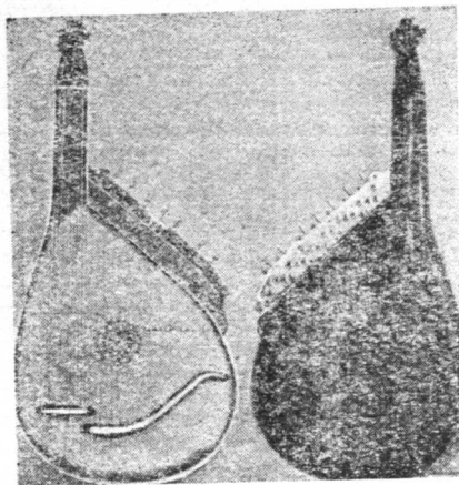
Бандура первого выпуска (лицевая и оборотная стороны) Черниговской музыкальной фабрики. Конструкция И. Скляра. Наверху механизм переключателя.
